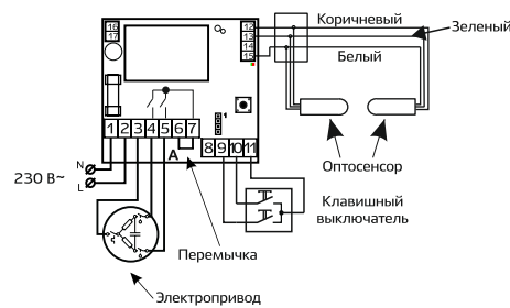
Рис. 2 — Подключение электропривода роллеты и оптоносенсора
