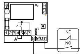
Рис. 3 — Подключение геркона
