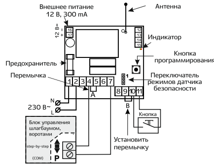
Рис. 1 — Подключение блока автоматики
